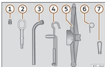
Fig. 213 En el maletero, bajo la cubierta de la superficie de carga: herramientas de a bordo.
