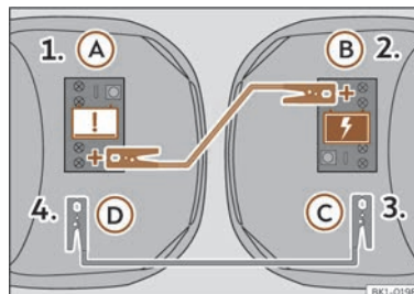
Fig. 216 Esquema de conexión de los cables de emergencia.
