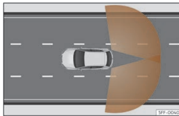
Fig. 134 Zonas de detección de los sensores.
