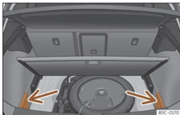
Fig. 183 En el maletero: tapas para guardar la bandeja.
