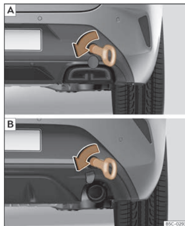
Fig. 222 En el lado derecho del paragolpes trasero: argolla de remolque enroscada. [A] Leon Sportstourer; [B] Leon.
