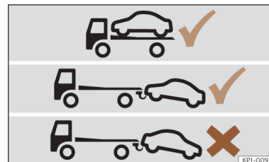
Fig. 217 Transportar con una grúa: vehículos con cambio automático y tracción delantera.
