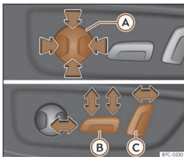
Fig. 96 Asiento del conductor: ajuste eléctrico del asiento.
