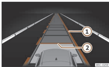
Fig. 147 En la pantalla del cuadro de instrumentos: visualización con la regulación activa (representación esquemática).
