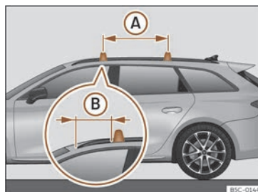
Fig. 202 Puntos de fijación de las barras transversales para el portaequipajes del techo (Leon Sportstourer).
