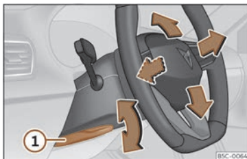
Fig. 94 Palanca en la parte inferior del lateral izquierdo de la columna de dirección.
