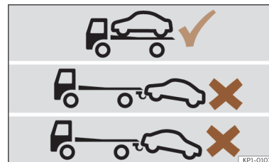
Fig. 218 Transportar con una grúa: vehículos con cambio automático y tracción total (4Drive).
