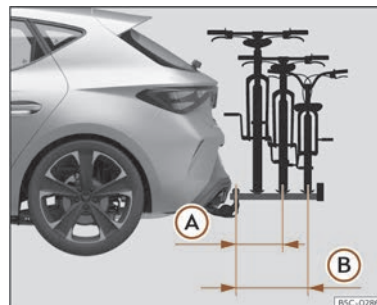
Fig. 207 Representación esquemática del voladizo máximo de la carga en un portabicicletas para dos o tres bicicletas.
