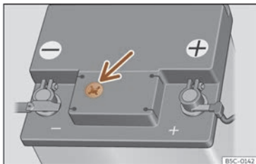
Fig. 239 Mirilla en la parte superior de la batería de 12 voltios (representación esquemática).
