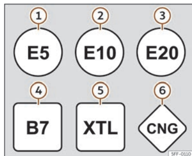
Fig. 211 Identificación de los combustibles según Directiva de la Unión Europea (UE) 2014/94/
