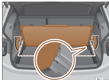
Fig. 138 En el maletero: fijar el segundo suelo del maletero.
