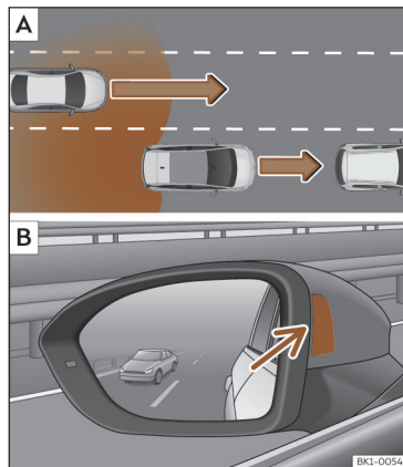
Fig. 113 Representación esquemática: A Situación en un adelantamiento con tráfico en la parte trasera. B Indicación del asistente de cambio de carril en el testigo de control del lado izquierdo.
