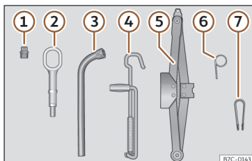
Fig. 143 En el maletero, bajo la cubierta de la superficie de carga: herramientas de a bordo.
