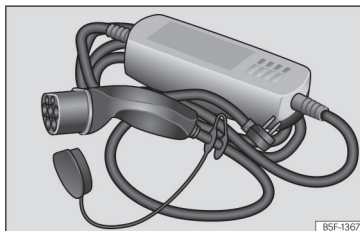
Fig. 54 Cable de carga para tomas de corriente.
