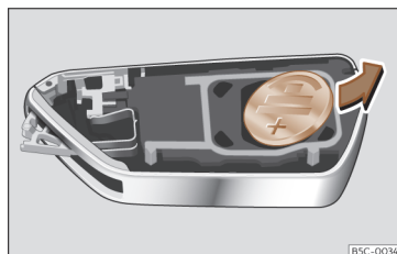
Fig. 59 Llave del vehículo: extracción de la pila.
