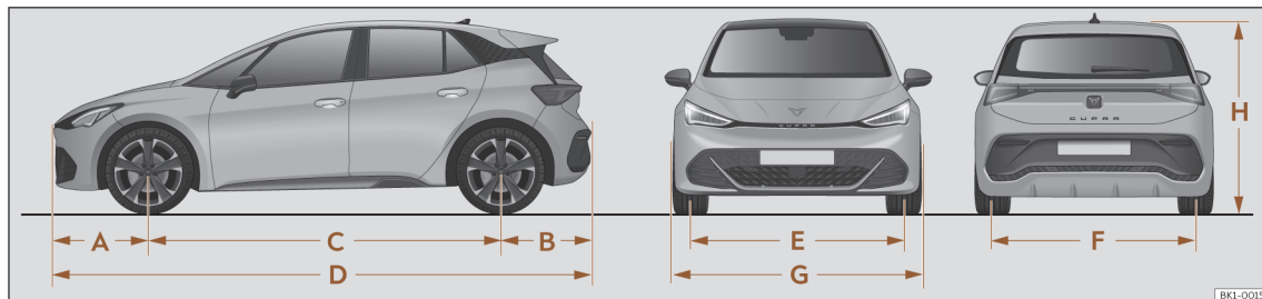
Fig. 171 Dimensiones
