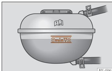
Fig. 157 En el vano delantero: marca en el depósito de expansión del líquido refrigerante.
