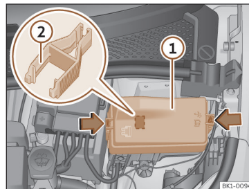
Fig. 153 En el vano delantero: tapa de la caja de fusibles.
