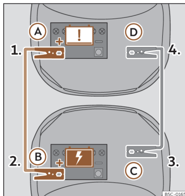
Fig. 148 Esquema de conexión de los cables de emergencia.
