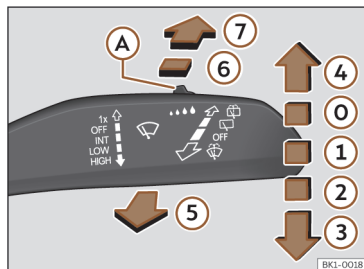
Fig. 85 Manejo del limpiaparabrisas y limpiaventana.
