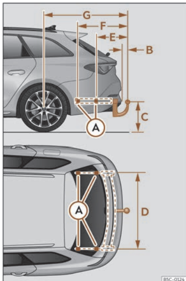
Fig. 202 Cotas e puntos de fixación para a montaxe posterior dun dispositivo de remolque.
