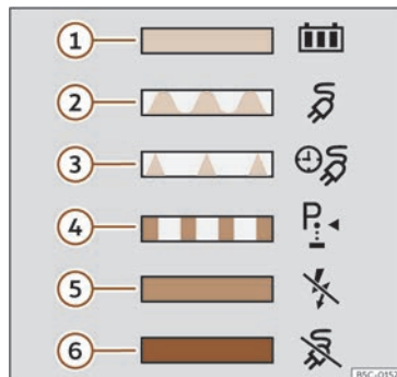
Fig. 209 Na cara interior da tapa da toma de carga da batería: adhesivo con información sobre o indicador do proceso de carga.
