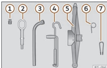
Fig. 38 No maleteiro, baixo a cuberta da superficie de carga: ferramentas de a bordo.
