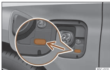
Fig. 208 Detrás da tapa da toma de carga da batería: indicador do proceso de carga.
