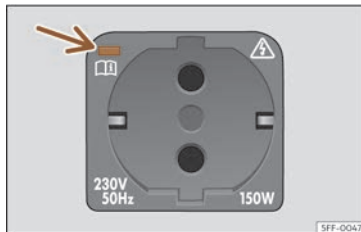
Fig. 144 No maleteiro: toma de corrente de 230 voltios.
