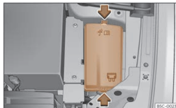
Fig. 53 No van motor: tapa da caixa de fusibles.
