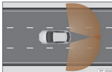
Fig. 166 Zonas de detección dos sensores
