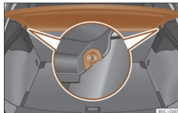
Fig. 118 No maleteiro: desmontar e montar a bandexa.
