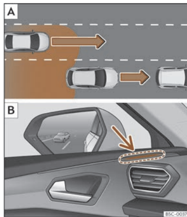
Fig. 184 Representación esquemática: A Situación nun adelantamento co tráfico na parte traseira. B Indicación do asistente de cambio de carril no indicador de control do lado esquerdo.
