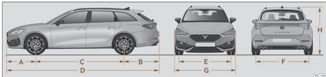
Fig. 240 Dimensions
