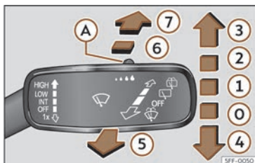
Fig. 103 Maneig de l'eixugaparabris- ses i eixugavidres posterior.
