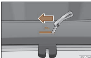
Fig. 79 Detall del maletger: desbloqueig d'emergència (Leon).
