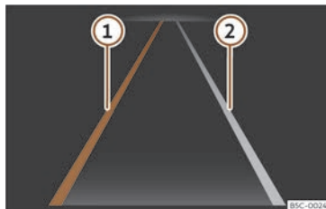
Fig. 137 A la pantalla del quadre d'instruments: indicacions del sistema d'avís de sortida del carril.
