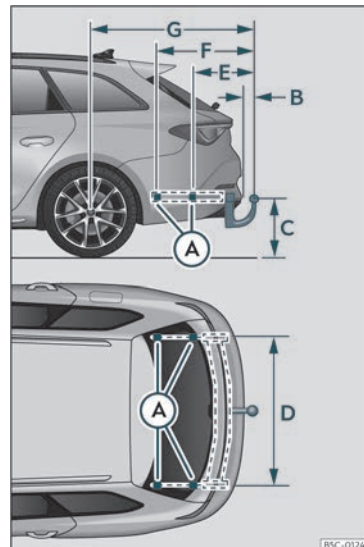
Fig. 199 Cotes i punts de fixació per al muntatge posterior d'un dispositiu de remolc.
