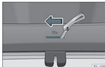
Fig. 89 Detall del maleter: desbloqueig d'emergència (Leon).
