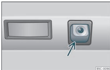
Fig. 164 Al para-xocs del darrere: ubicació de la càmera de l'assistent per a marxa enrere.
