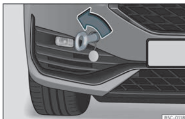
Fig. 48 Part dreta del para-xocs davanter: argolla de remolc enroscada.
