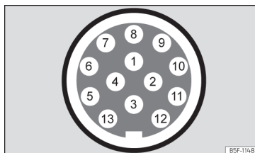
Fig. 197 Representació esquemàtica::assignació dels pins de la presa de corrent per a remolc.
