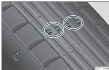
Fig. 224 Perfil del pneumàtic: Indicadors de desgast.
