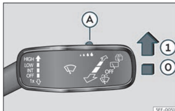
Fig. 100 Palanca de l'eixugaparabrises: ajustar el sensor de pluja (A)
