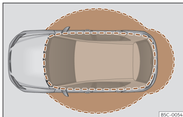
Fig. 68 Keyless Access: zonas de proximidad.
