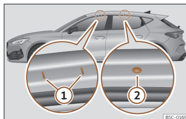
Fig. 193 Puntos de fijación de las barras longitudinales para el portaequipajes del techo (Leon).
