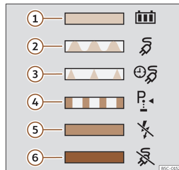
Fig. 58 En la cara interior de la tapa de la toma de carga de la batería: adhesivo con información sobre el indicador del proceso de carga.
