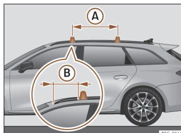
Fig. 192 Puntos de fijación de las barras longitudinales para el portaequipajes del techo (Leon Sportstourer).
