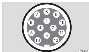
Fig. 194 Representación esquemática: asignación de los pines de la toma de corriente para remolque.
