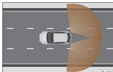
Fig. 125 Zonas de detección de los sensores.
