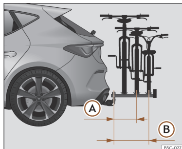
Fig. 197 Representación esquemática del voladizo máximo de la carga en un portabicicletas para dos o tres bicicletas.
