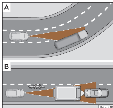
Fig. 132 A) Vehículo en una curva. B) Motociclista circulando por delante fuera del radio de acción del sensor de radar.
