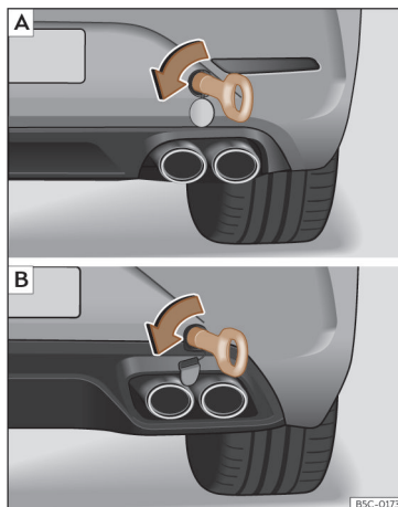
Fig. 209 En el lado derecho del paragolpes trasero: argolla de remolque enroscada. A Leon Sportstourer; B Leon.
