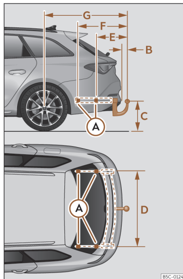
Fig. 198 Cotas y puntos de fijación para el montaje posterior de un dispositivo de remolque.
