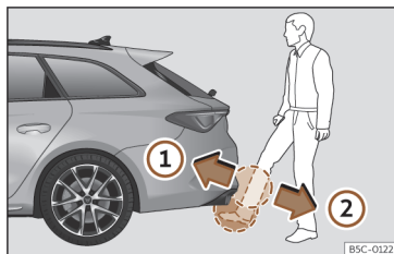
Fig. 78 Portón del maletero con apertura controlada por sensor (Easy Open).
