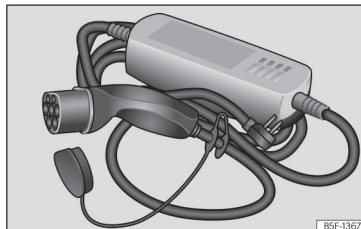
Fig. 61 Cable de carga para tomas de corriente.
