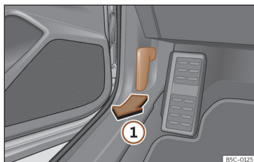
Fig. 217 Palanca de desbloqueo en el espacio reposapiés del conductor.
