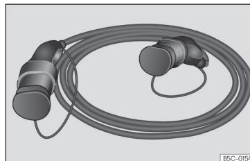
Fig. 211 Cable de carga para estaciones de carga con corriente alterna (CA).
