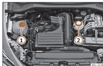
Fig. 224 Vano motor: Depósitos de líquido refrigerante
