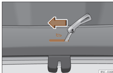
Fig. 91 Detalle del maletero: desbloqueo de emergencia (Leon).
