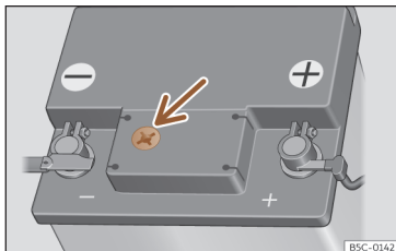
Fig. 230 Mirilla en la parte superior de la batería de 12 voltios (representación esquemática).
