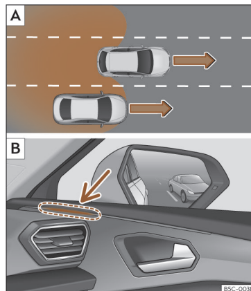
Fig. 185 Representación esquemática: [A] Situación en un adelantamiento en el carril central e incorporación posterior al carril derecho. [B] Indicación del asistente de cambio de carril en el testigo de control del lado derecho.
