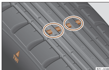
Fig. 232 Perfil del neumático: indicadores de desgaste.
