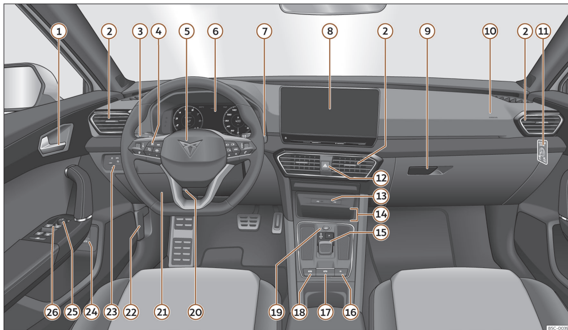
Fig. 55 Puesto de conducción.
