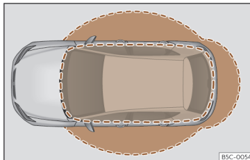
Fig. 82 Keyless Access: zonas de proximidad.
