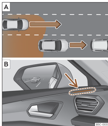
Fig. 184 Representación esquemática: [A] Situación en un adelantamiento con tráfico en la parte trasera. [B] Indicación del asistente de cambio de carril en el testigo de control del lado izquierdo.
