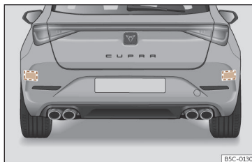
Fig. 165 Vista trasera del vehículo: zonas de los sensores de radar.
