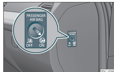
Fig. 19 Conmutador con llave para activar y desactivar el airbag del acompañante.
