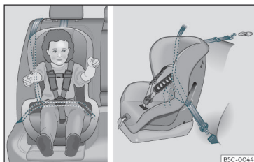
Fig. 35 En los asientos traseros: montaje del asiento para niños.
