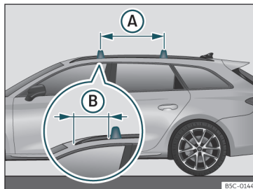
Fig. 136 Puntos de fijación de las barras longitudinales para el portaequipajes del techo (Leon Sportstourer).
