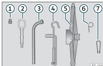
Fig. 37 En el maletero, bajo la cubierta de la superficie de carga: herramientas de a bordo.
