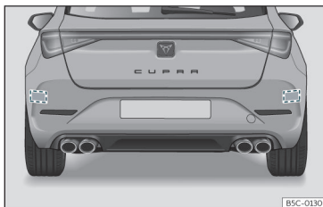
Fig. 162 Vista trasera del vehículo: zonas de los sensores de radar.
