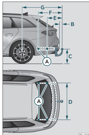
Fig. 199 Cotas y puntos de fijación para el montaje posterior de un dispositivo de remolque.
