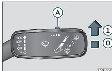
Fig. 100 Palanca del limpiaparabrisas: ajustar el sensor de lluvia (A).
