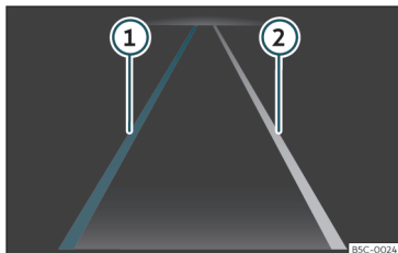
Fig. 175 En la pantalla del cuadro de instrumentos: indicaciones del sistema de aviso de salida del carril.
