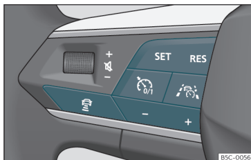
Fig. 178 Lado izquierdo del volante multifunción: teclas para el manejo del Travel Assist.
