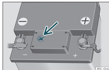
Fig. 221 Mirilla en la parte superior de la batería de 12 voltios (representación esquemática).
