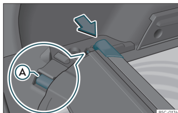
Fig. 121 En el maletero: alojamiento para guardar la bandeja enrollable.
