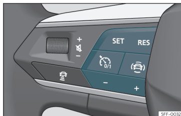
Fig. 166 En el volante multifunción: botones para manejar el limitador de velocidad
