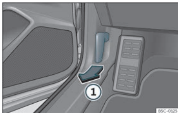
Fig. 183 Panca de desbloqueo no espazo repousapés do condutor.
