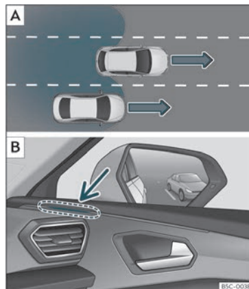
Fig. 163 Representación esquemática: [A] Situación nun adelantamento no carril central e incorporación posterior ao carril dereito. [B] Indicación do asistente de cambio de carril no indicador de control do lado dereito.
