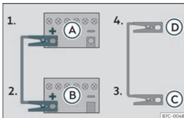
Fig. 42 Esquema de conexión para vehículos con sistema Start-Stop.
