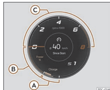
Fig. 56 Quadre d'instruments digital: Powermeter (vista clàssica)
