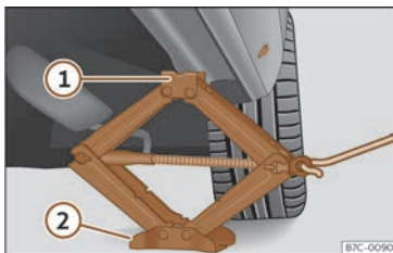
Fig. 39 Llanguer: col·locació del gat del vehicle.
