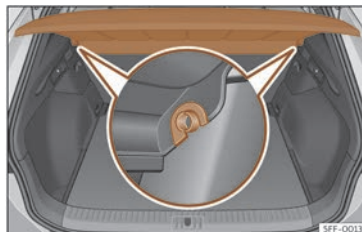
Fig. 112 Al maleter: desmuntar i muntar la safata.
