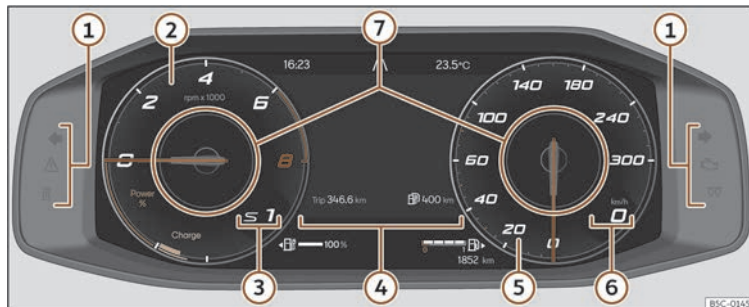
Fig. 52 Digital Cockpit al tauler d'instruments (vista clàssica).
