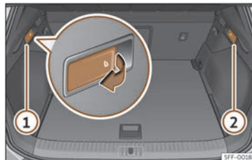
Fig. 109 Al maleter: palanques per al desbloqueig del respatllet del darrere.
