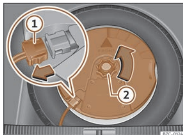
Fig. 224 Al maleter: desmuntar el subwoofer.
