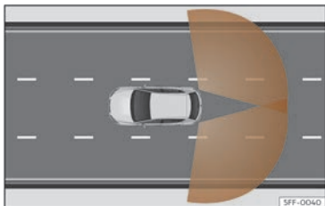
Fig. 152 Zones de detecció dels sensors
