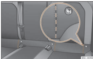
Fig. 27 Seient posterior: ranures encunades per accedir a les anelles de subjecció ISOFIX/i-Size.
