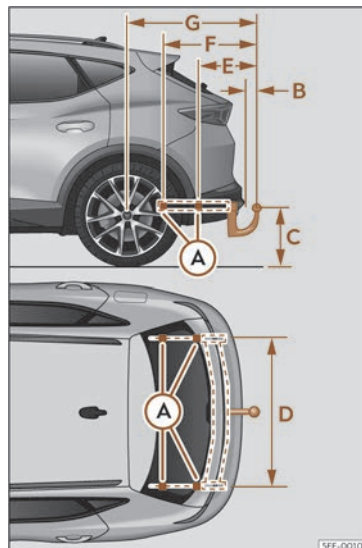
Fig. 189 Cotes i punts de fixació per al muntatge posterior d'un dispositiu de remolc.
