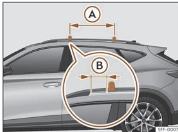
Fig. 123 Punts de fixació de les barres longitudinals per al portaequipatges del sostre.
