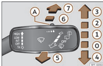
Fig. 96 Maneig de l'eixugaparabrises i eixugavidres posterior.
