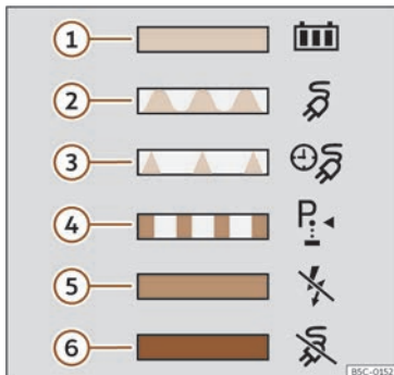
Fig. 196 A la cara interior de la tapa de la presa de càrrega de la bateria: adhesiu amb informació sobre l'indicador del procés de càrrega.
