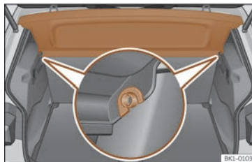
Fig. 169 No maleteiro: desmontar e montar a bandexa.
