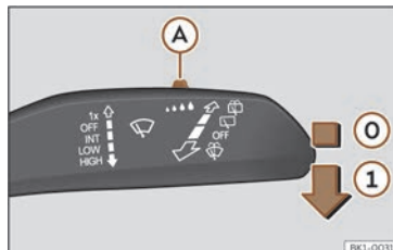
Fig. 108 Panca do limpaparabrisas: axustar o sensor de choiva A .
