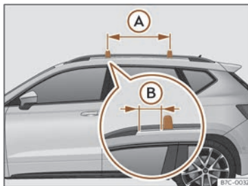
Fig. 118 Punts de fixació de les barres longitudinals per al portaequipatges del sostre.
