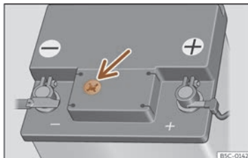
Fig. 203 Espiall a la part superior de la bateria de 12 volts (representació esquemàtica).
