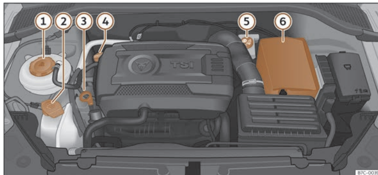
Fig. 194 Figura orientativa de la posició dels elements.
