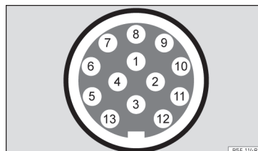
Fig. 187 Representació esquemàtica:: assignació dels pins de la presa de corrent per a remolc.
