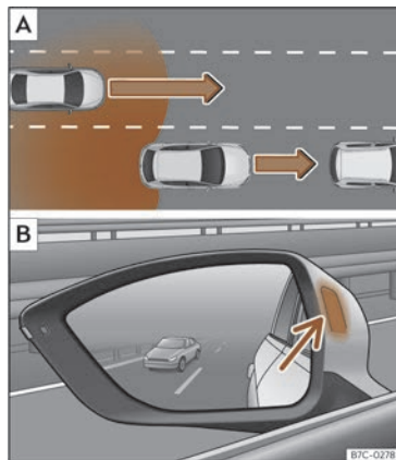
Fig. 165 Representació esquemàtica: [A] Situació en un avançament amb trànsit a la part posterior. [B] Indicació de l'assistent de canvi de carril al retrovisor exterior esquerre.
