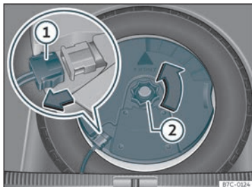
Fig. 269 Al maleter: desmuntar el subwoofer.
