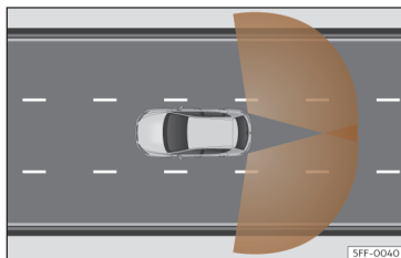
Fig. 147 Zonas de detección de los sensores
