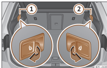
Fig. 103 En el maletero: palancas para desbloqueo a distancia de las partes izquierda ① y derecha ② del respaldo trasero.
