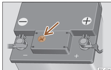
Fig. 203 Mirilla en la parte superior de la batería de 12 voltios (representación esquemática).
