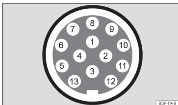
Fig. 187 Representación esquemática: asignación de los pines de la toma de corriente para remolque.
