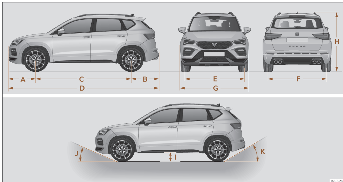
Fig. 210 Dimensiones y ángulos.
