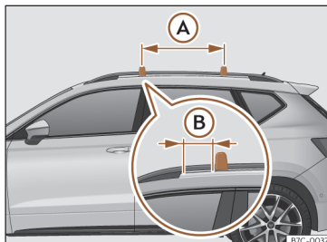
Fig. 118 Puntos de fijación de las barras longitudinales para el portaequipajes del techo.
