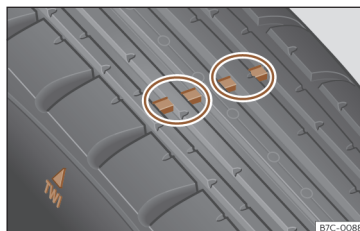
Fig. 205 Perfil del neumático: indicadores de desgaste.
