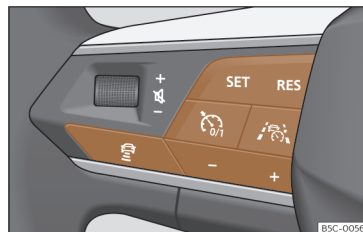
Fig. 162 Lado izquierdo del volante multifunción: teclas para el manejo del Travel Assist.
