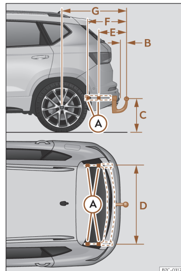
Fig. 189 Cotas y puntos de fijación para el montaje posterior de un dispositivo de remolque.
